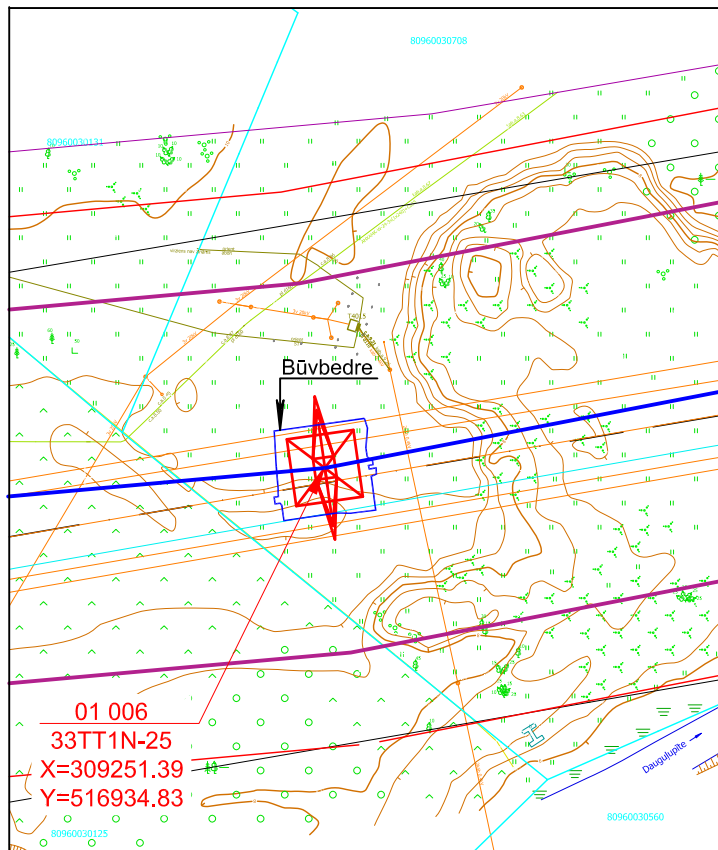
Balsta Nr. 01 006 būvbedres novietojums topogrāfiskajā plānā (M ~)
